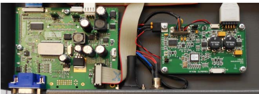
Das Bedienpanel des TFT-Displays ist auf einem Geräteträger vormontiert.
